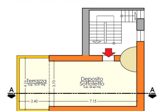
Situazione in Variante PIANTA PIANO TERZO
